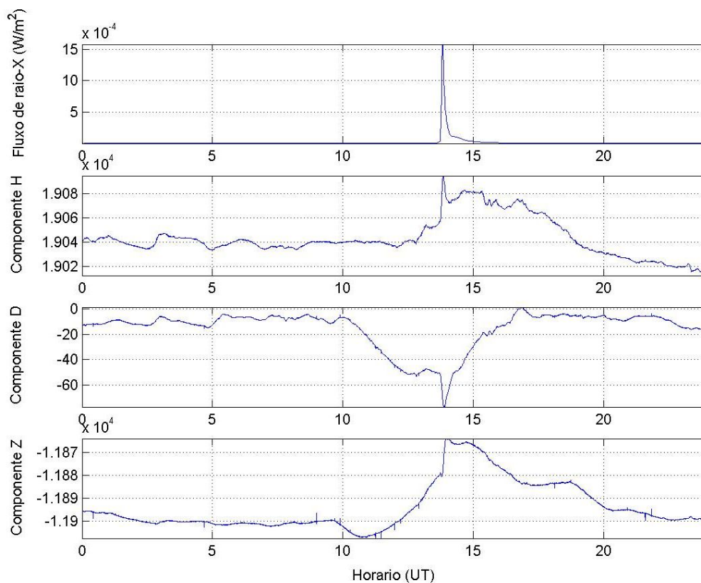
Figura 6.4 – Dados obtidos dos Satélites GOES e dos Magnetômetros do Observatório Espacial de Sul – OES/CRS/INPE – MCT, em São Martinho da Serra, RS, para o dia 15 de abril de 2001.
